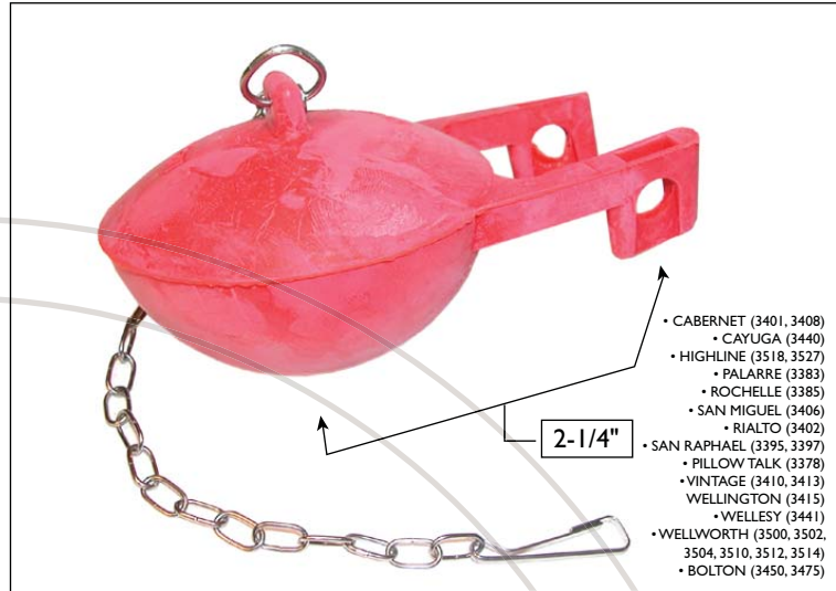
KOH49114 • FLAPPER
